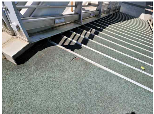
계단부 P1 투수콘 파손
