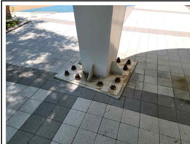
계단부 P1 볼트부식
